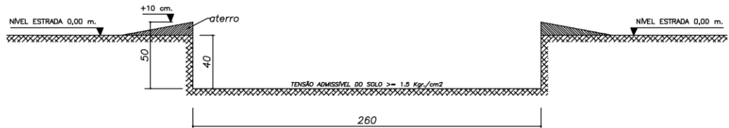
VISTA ESCAVAÇÃO LATERAL
