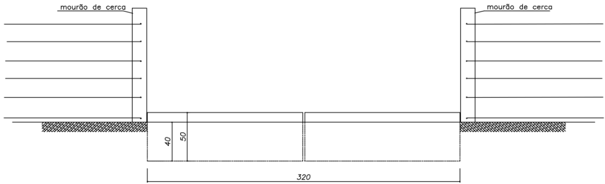
VISTA COLOCAÇÃO FRONTAL
