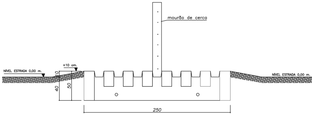
VISTA COLOCAÇÃO LATERAL
